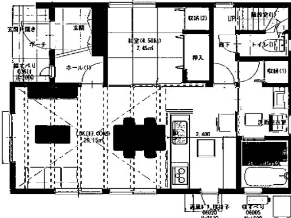
1階平面図
